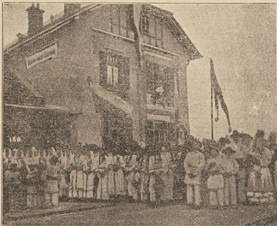
K otvoritvi belokranjske železnice: Beli Kranjci v narodni noši na črnomaljskem kolodvoru.
