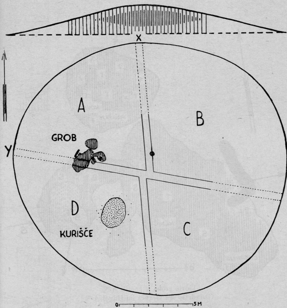
Profil in tloris gomile A-3 Profil und Grundriss des Hügelgrabes A-3
