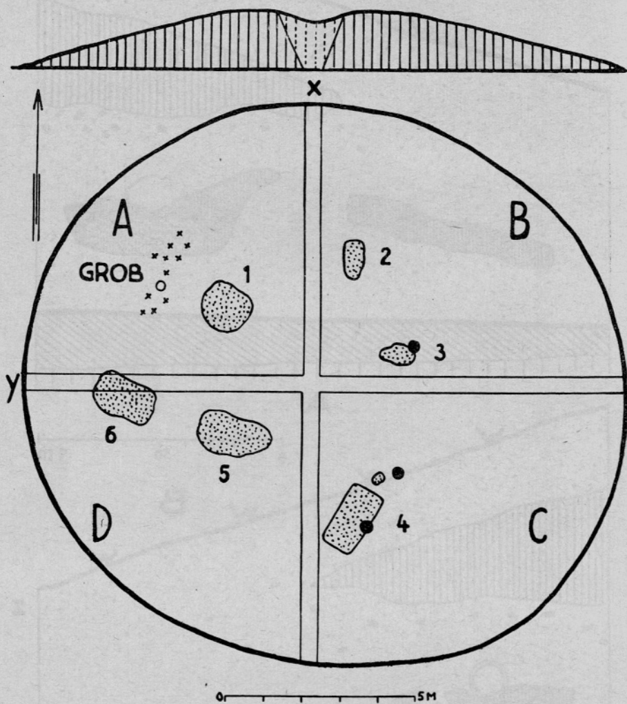
Profil in tloris gomile A-4 Profil und Grundriss des Hügelgrabes A-4
