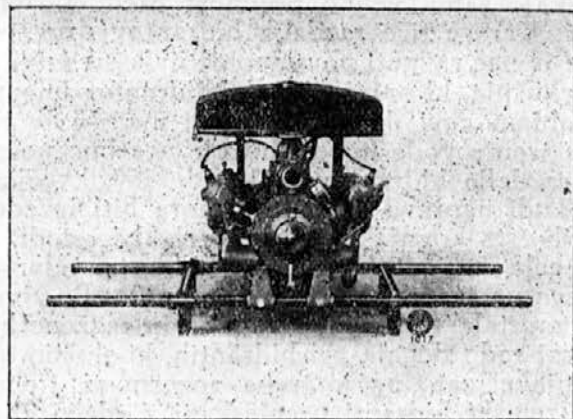
Nosna lahka, motorna brizgalnica.
