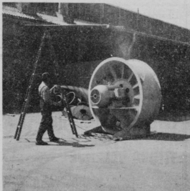
Barvanje velikega aksialnega ventilatorja
