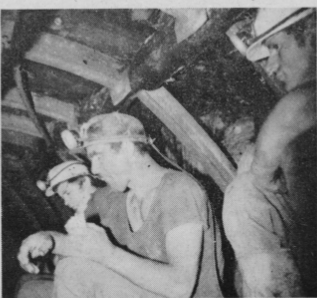
Jeklena konstrukcija jamskega oporja je sodobnejša, vendar je tu postavljeno dodatno pred lesen opaž.
