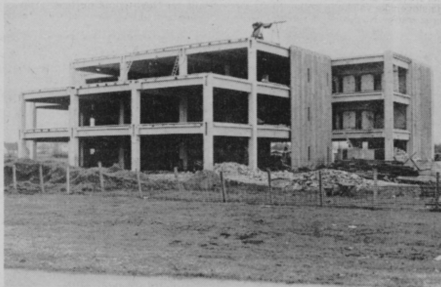
Takole gradijo Ingradovci v Živinicah pri Tuzli novo trgovsko hišo po montažnem sistemu armirane betonske konstrukcije v treh etažah.
