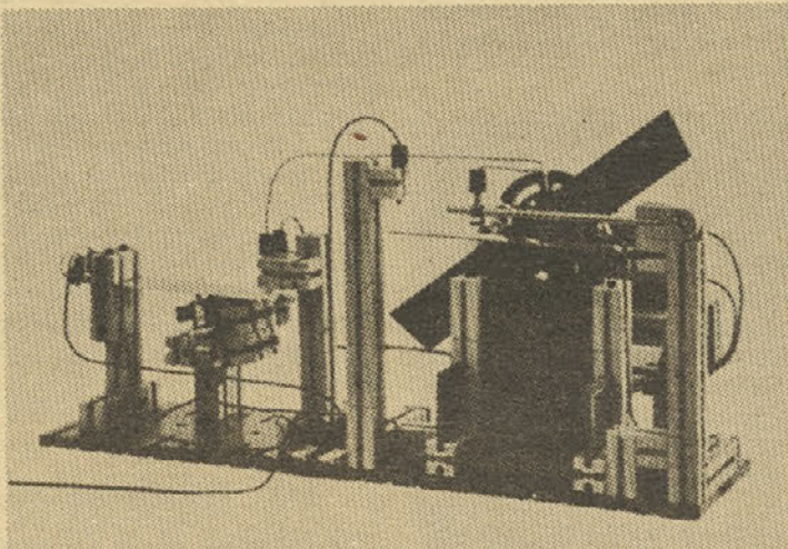
Demonstracijski model avtomatičnega uravnavanja klimatske naprave s termostatom in regulatorjem.
