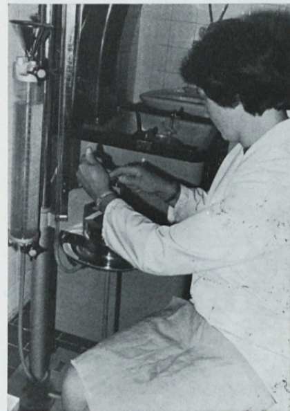
Schopper aparat za preizkušanje vodonepropustnosti
