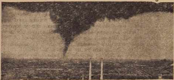
Orkan se je približeval z blazno naglico. Značilen je ogromnemu lijaku podoben vrtnec na sliki
