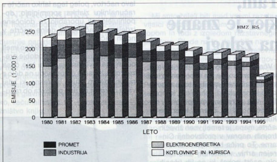
Emisija SO 2 v Sloveniji, 1980 - 1995
