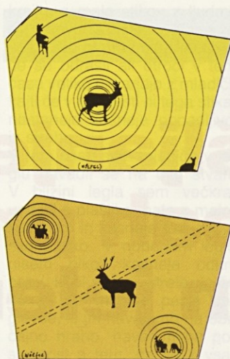
Shematični prikaz razlike v vidiku teritorialnosti pri srnjaku in pri jelenu.
