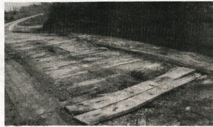
Slika nam prikazuje most čez vodo »Bistrice« v Bistri. Cesta pa pelje iz Bistre proti hlevom Ljubljanskega posestva in na različna privatna zemljišča. Kot se vidi, je most potreben takojšnjega popravila vrhnega ustroja, da ne bo prišlo do kakšne katastrofe. (S.S.)
