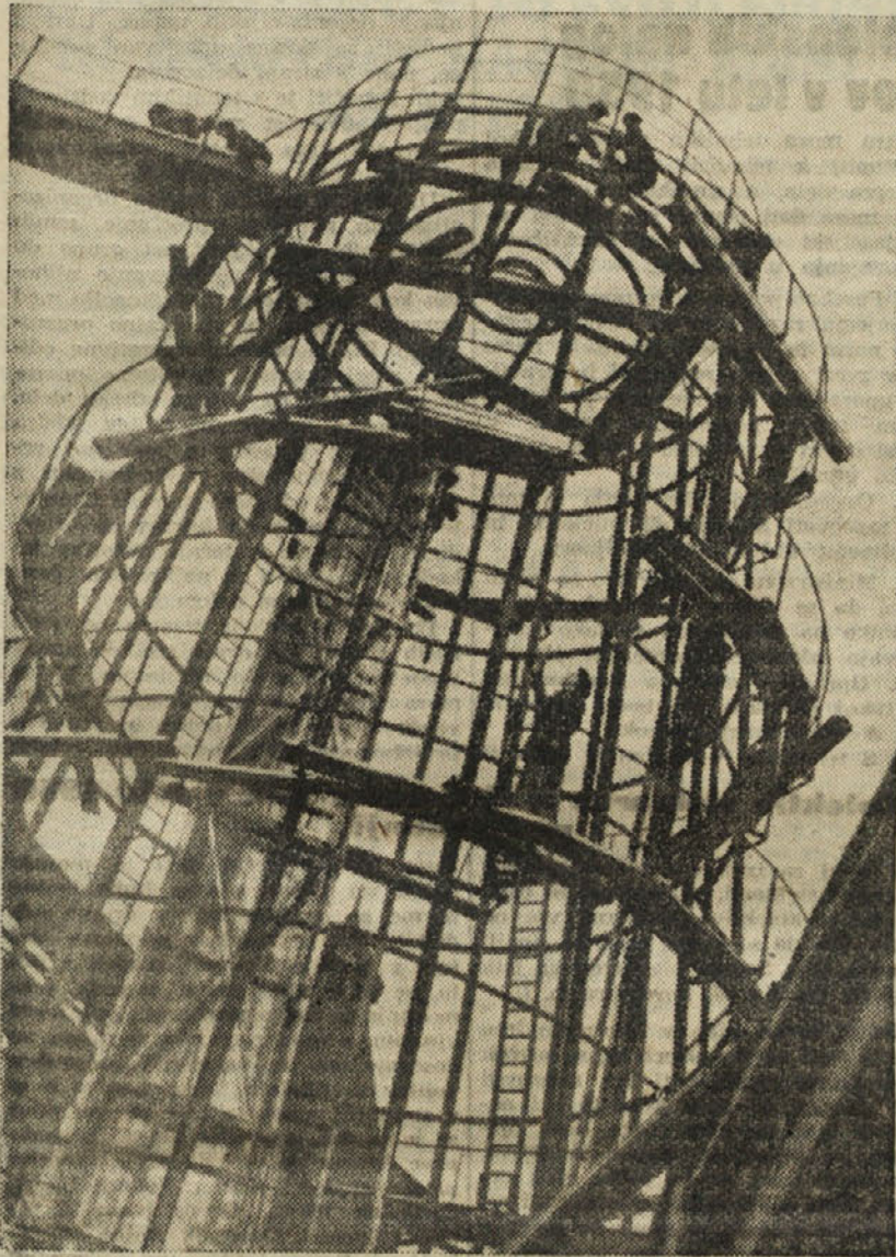
Zelesno ogrodje za novo 15 m visoko Mills-Packardovo komoro v tovarni kemičnih izdelkov v Hrastniku
