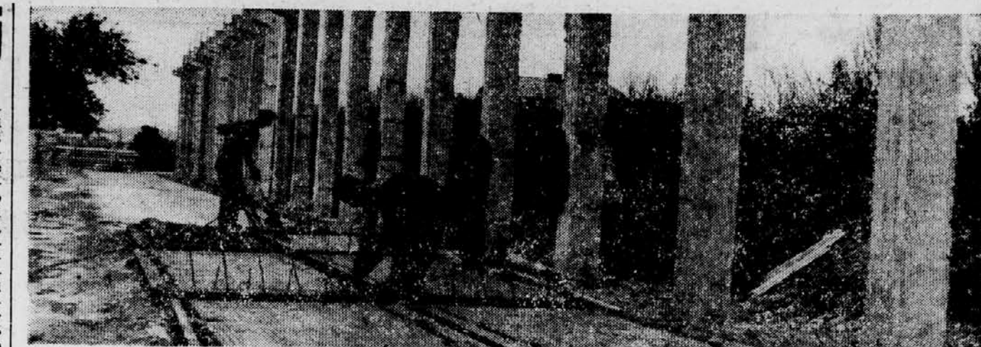
MONTAŽNI DELI ZA 500 STANOVANJ — Celjsko industrijsko gradbeno podjetje, ki se je preteklo leto v velikem obsegu lotilo popolnoma montažne gradnje stanovanj, ima ob Savinji docela mehaniziran obrat za proizvodnjo sestavnih delov. Vsega 20 delavcev, delovodja in skladiščnik izdelajo v 1 letu sestavne dele za 500 družinskih stanovanj. Dovoz betonske mehanice, oblikovanje montažnih delov, prekladanje letih in ves nadaljnji transport so mehanizirali. Do zime bo izdelovalnica montažnih stanovanjskih delov ob Savinji v Celju dobila še streho in okna, tako da bo proizvodnja stanovanj »na zalogo« nemoteno tekla tudi v zimskem času.
