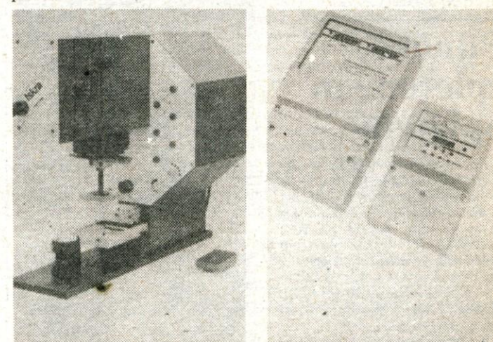
Profesionalna naprava za tiskanje s tamponom TAMPOTISK TT 100.
