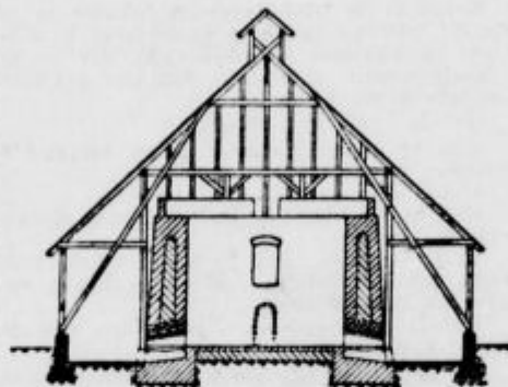
Sl. 17b. Poljska peč za žganje opeke. Prečni prerez A-A.
