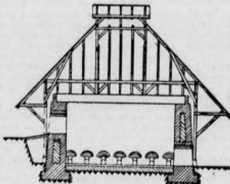
Sl. 17c. Vzdolžni prerez B-B.
