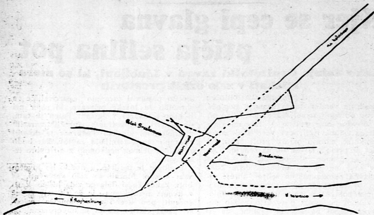
Železobetonski most čez potok Brestanica v Rajhenburgu na banovinski cesti II/159. Situacija: M 1:500.
