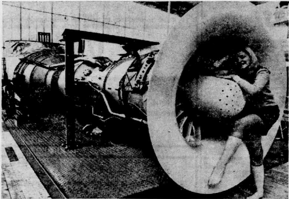
STROJI IN OPREMA ZA LADJE — Posebnost letošnjega pomorskega sejma v Hamburgu je bila osem ton težka ladijska plinska turbina s 30.000 konjskimi močmi, izdelana pri Boeingu v ZDA (na sliki). Med drugim so pokazali računalniške za krmilo na velikih tankerjih, žaromete z dosegom šest kilometrov, majhne petrolejke za kabine pa posteljo, ki se tako ziblje, da potnik ne čuti nihanja ladje zaradi visokih valov.
