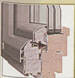
Nizkoenergijsko les-aluminij okno
