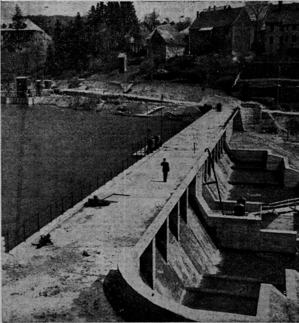
Cez pregrado umetnega jezera Bajer so speljali cesto do Fužin. Ob jezeru (na levi strani slike) je majhna hišica za avtomatno čiščenje vode. S tega mesta odteka voda po 10 km dolgi poti skozi predor pod Fužinami, cevodov Ličko polje, predor Kobiliak — Razomir in jelski tunel cevodov do 660 metrov nize ležeč podzemeljske strojnice v Triblju nad Crikvenico.
