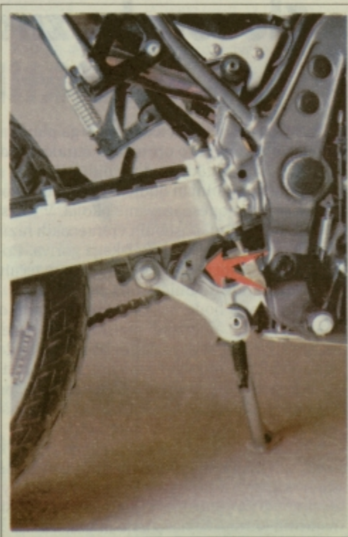
Preprost sistem vpetja zadnjega blažilnika dovoljuje znižanje motocikla za 4 cm.
