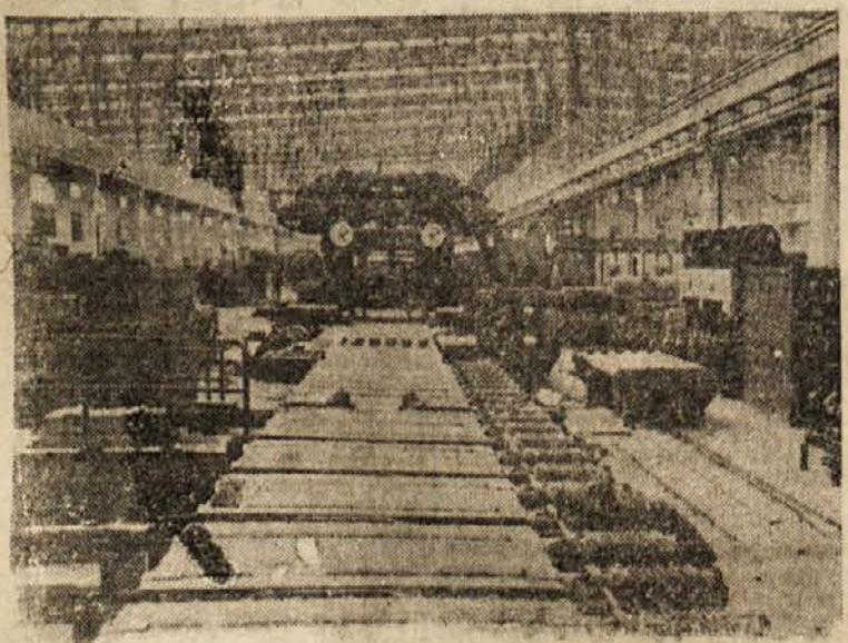
Kakor smo že poročali, bo začela v kratkem poskusno obratovati nova valjarna bakra v Sevojnem. Na sliki vidimo del notranjosti.
