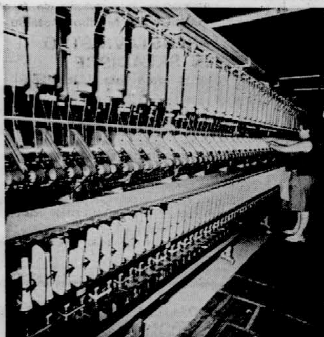
Novi predilni stroji za predenje kemijskih vlaken
