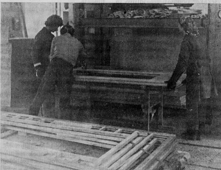
Pri lepljenju vhodnih in garažnih vrat v Mojstrani se oblogo pritrdi na skelet s sponkami, tako da ne pride do premika v stiskalnici
