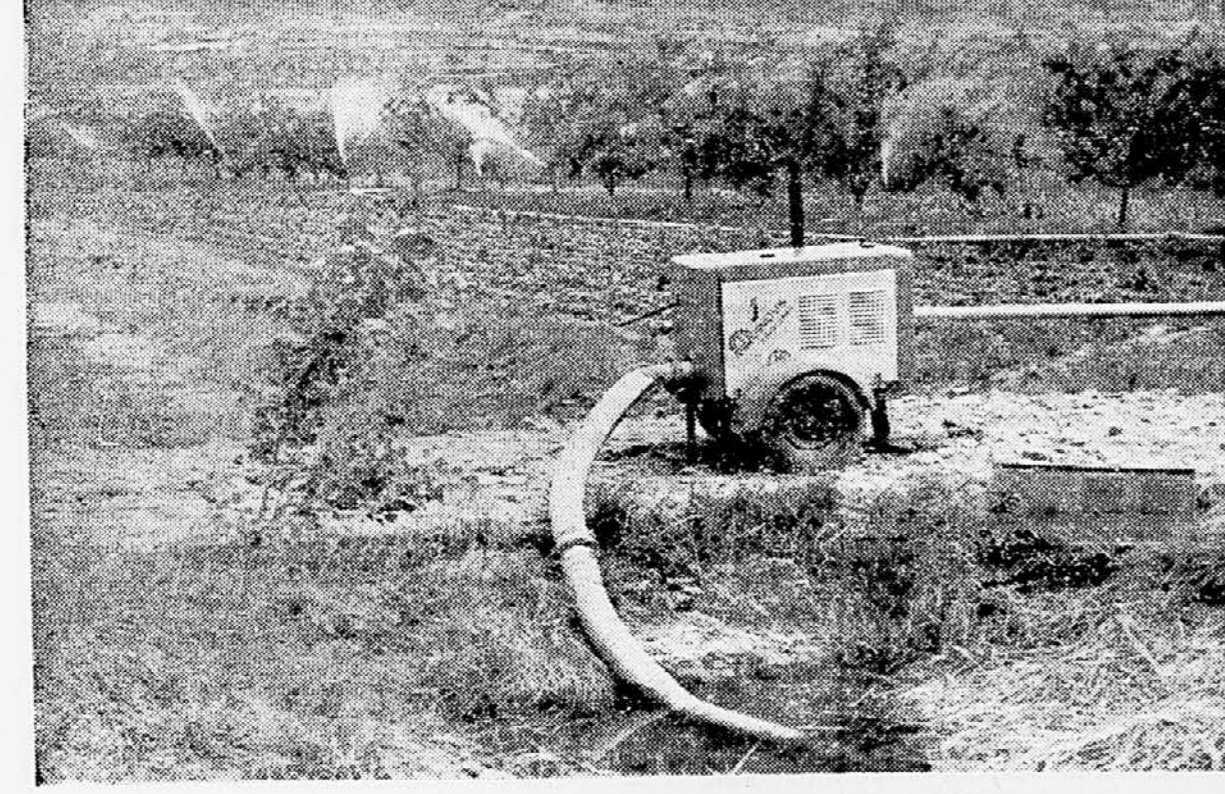
Letošnja spomladanska suša bi pridelovalcem s posestva Skočjan pri Kopru prizadejala precejšnjo škodo, če jo ne bi le-ti pričakali pripravljani. Oskrbeli so se namreč z agregatom tovarne Agrolindus za umetno namakanje, ki ga vidimo na sliki. Ko smo posestvo obiskali, je bil agregat v polnem pogonu in je razprševal vodo skozi 18 razpršilcev. Znal pa je tudi, da pravilno in izdatno zagonejene kulture mnogo bolje prenašajo sušo, zato so se uspešno poslužili tudi tega načina obrambe proti suši (foto Svabič)
