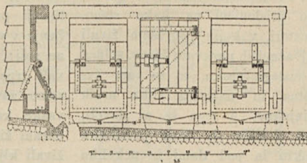
Slika d in e . Stena hodnika s kanalom v počeznem in podolžnem prerezu.
