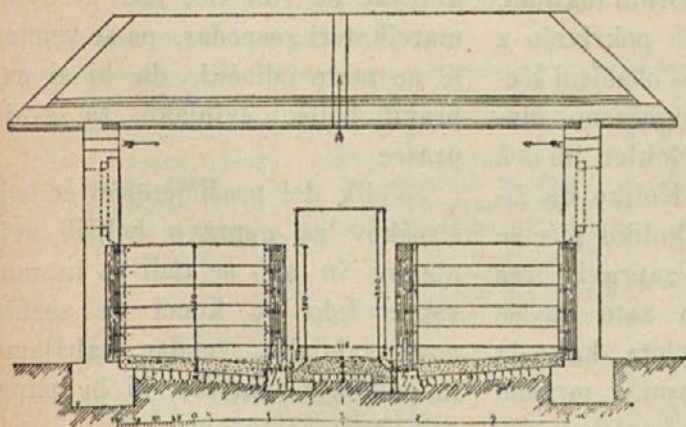
Slika c . Prerez CD svinjaka.
