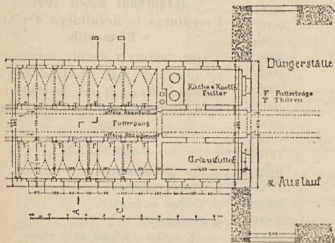
Slika a . Tloris svinjaka.
