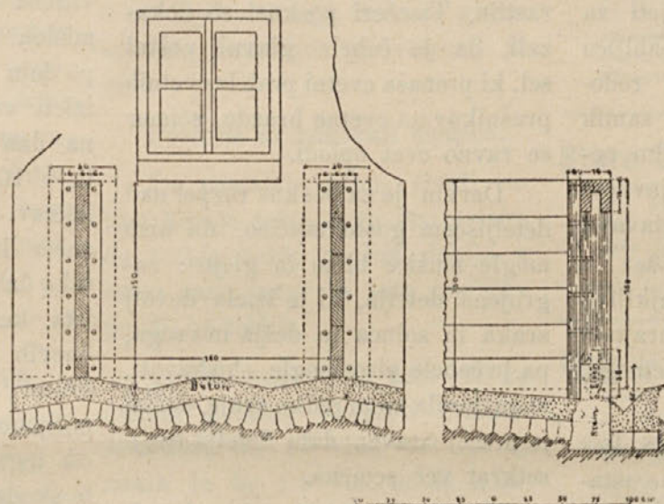
Slika f. Prerez enega prostora.
