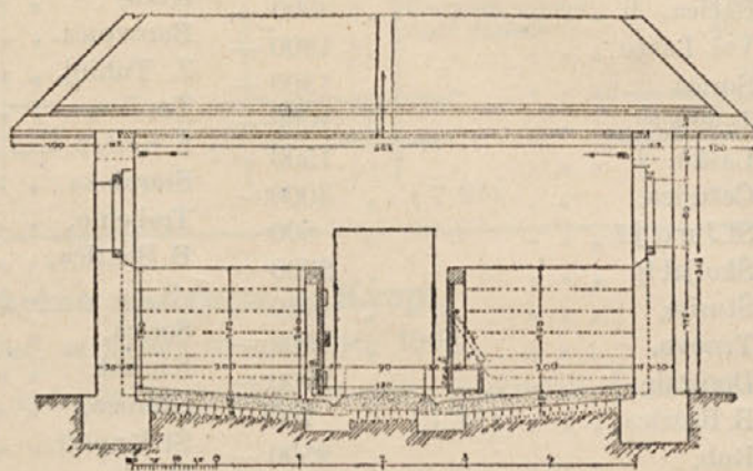
Slika b . Prerez AB svinjaka.
