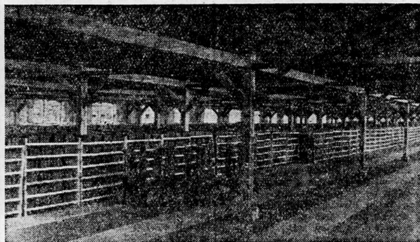
Sodobno urejen opekarški obrat v Gornji Radgoni. V sušilnih lopah so vrste surovega zidaka, ob njih pa avtomatizirani vozčki, s katerimi so precej mehkanizirali odlaganje surovega zidaka v sušilnice.
