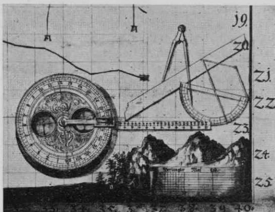
Steinbergovi merilni instrumenti (Detajl z originala, ki ga hrani Arhiv dvorne komore, Dunaj, Zbirka kart, signatura P c 1)
