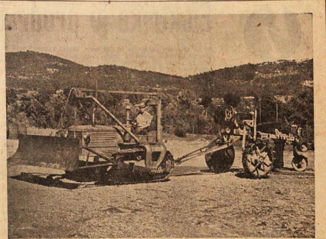
Garnitura za rigolanje vinogradov
