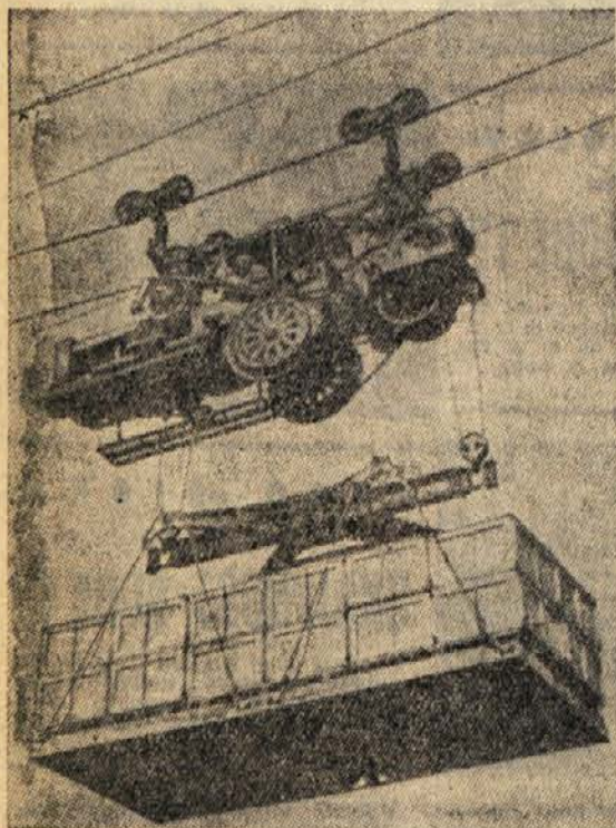
Na sliki vidite zračno železnico, ki jo uporabljajo v ZDA za iztovarjanje in natovarjanje ladij
