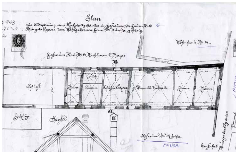
Adaptacijski načrt Plečnikove rojstne hiše l. 1896 (Vir: Zgodovinski arhiv Ljubljana)
