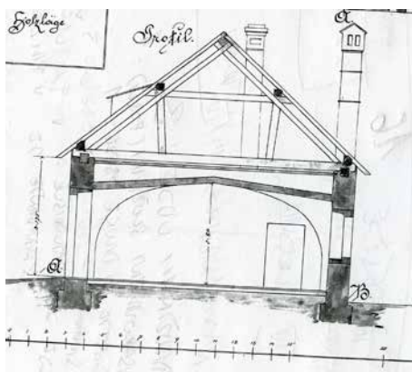
Adaptacijski načrt Plečnikove rojstne hiše l. 1896 (Vir: Zgodovinski arhiv Ljubljana)
