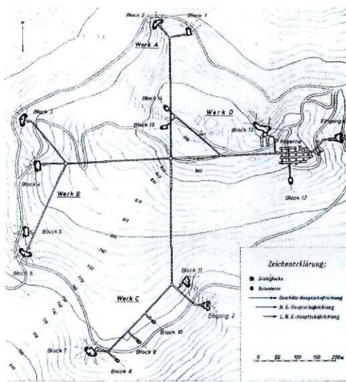
Ena izmed mnogih skic v knjigi; načrt za nedokončan utrdbeni sistem na Vrhju Svetih Treh Kraljev
