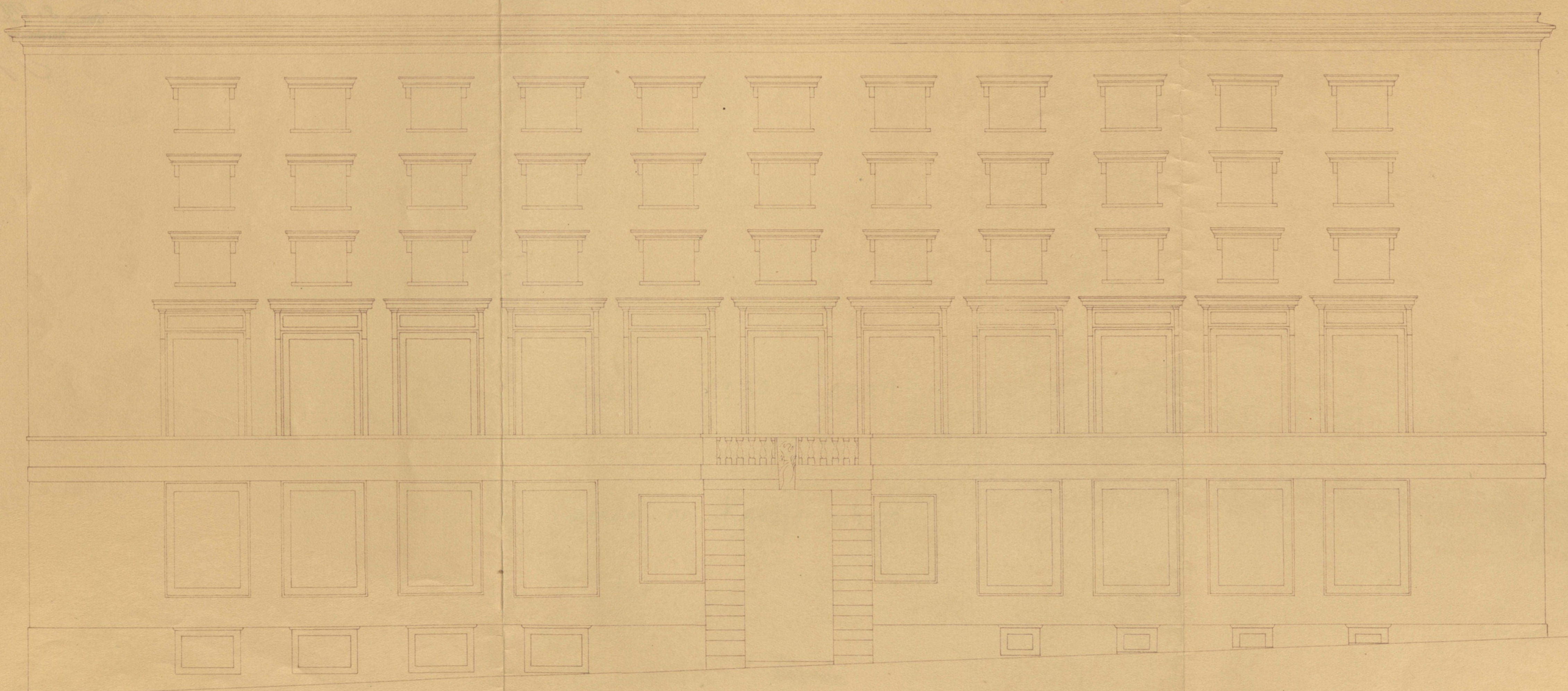
FASADA NA KNEŽJO ULICO
