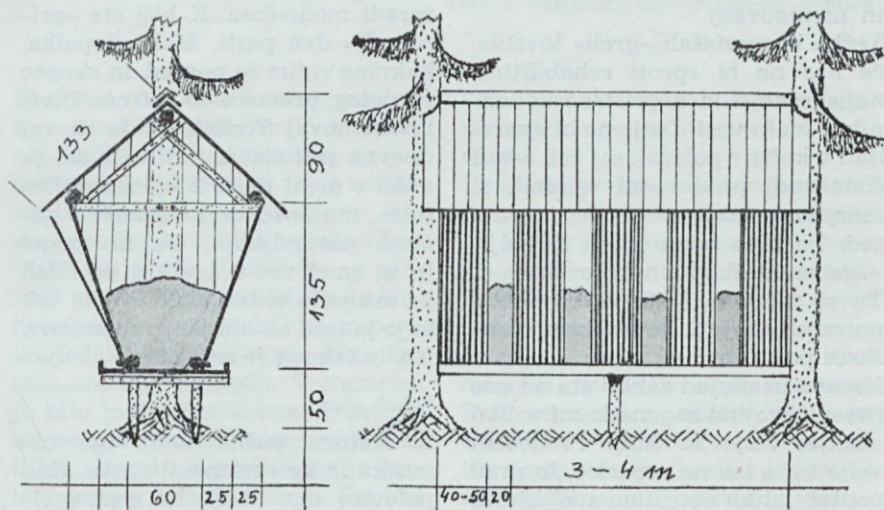
Krmilnica za gamse, srnjad in jelenjad, v prerezu in od strani
