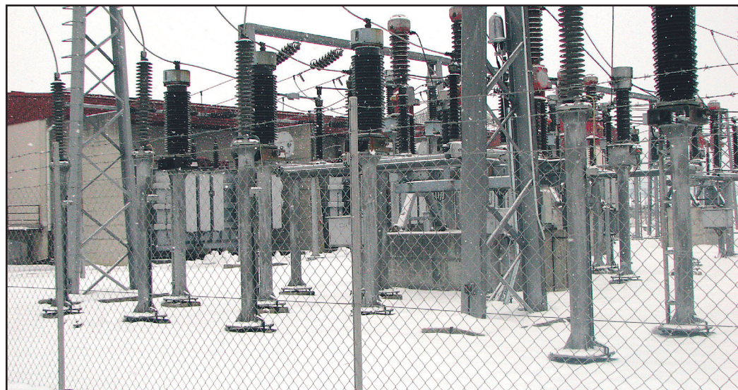
Razdelilna transformatorska postaja v Pesju
