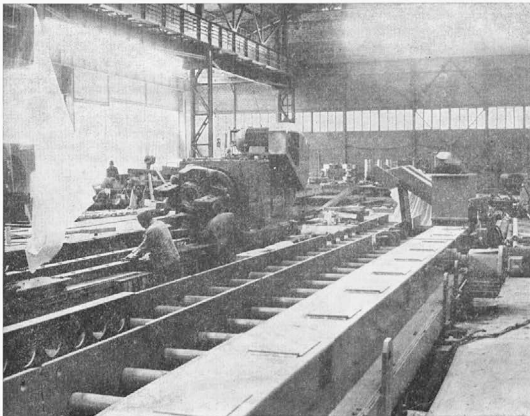
Montaža avtomatskega kovaškega stroja, september 1979
