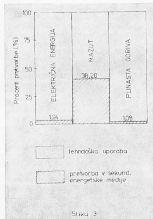
Slika 3 Stopnja direktne pretvorbe primarnih energetskih medijev v sekundarne v železarni Ravne
