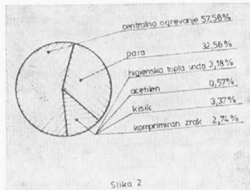
Slika 2 Struktura sekundarnih energetskih medijev v železarni Ravne v letu 1978
