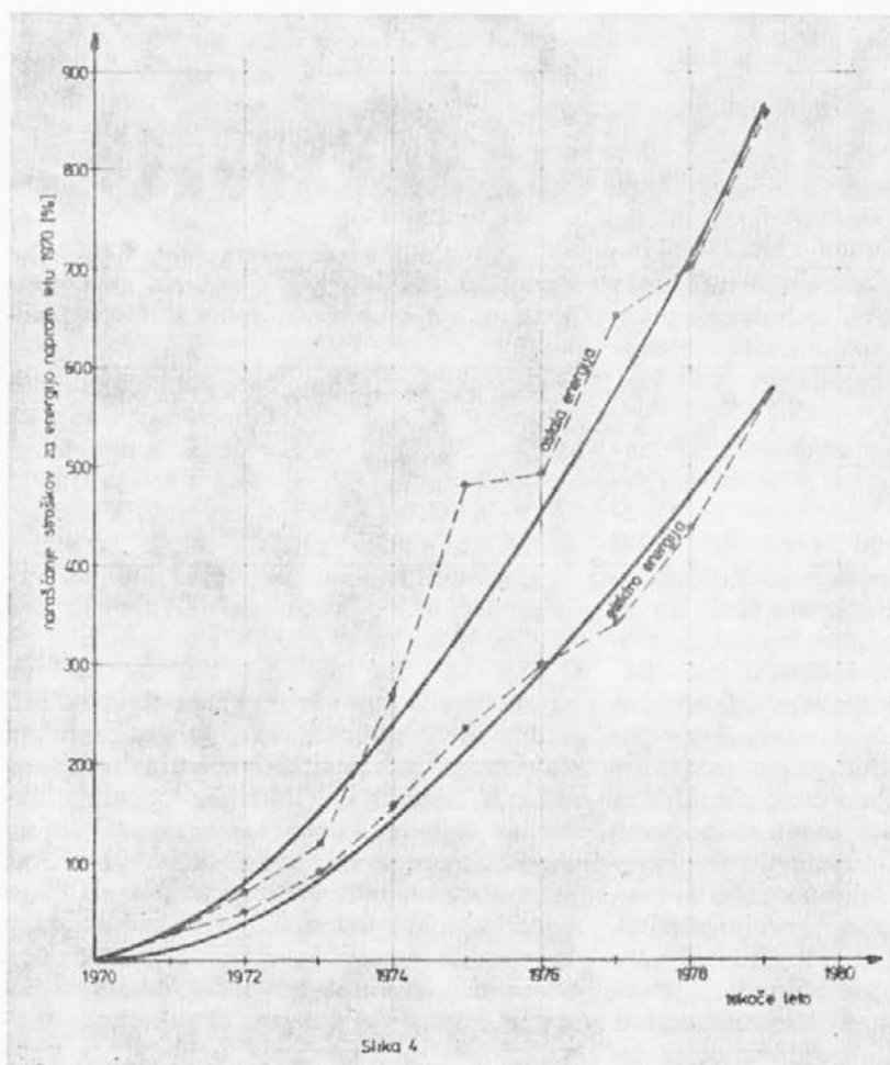
Porast cene toplotne energije na enoto proizvedenega jekla v železarni Ravne za obdobje 1970 do 1979
