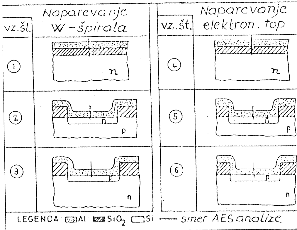
Slika 1: Shematski prikaz prereza vzorcev
