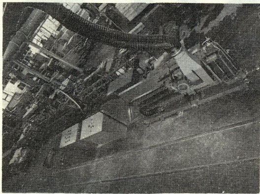
Linija za dolžinsko spajanje lesa tip HK 400, postavljena v decimirci v TOZD Mojstrana (pogled od zgoraj)
