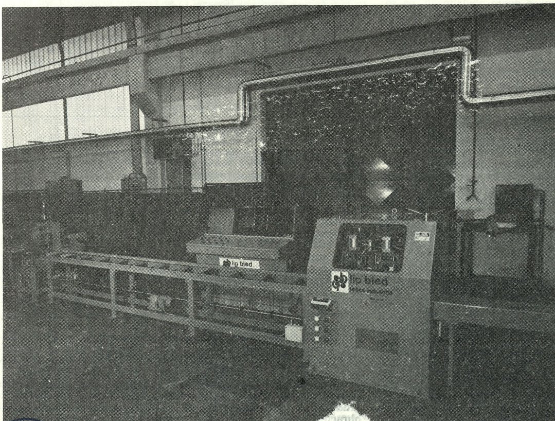
Linija za dolžinsko optimiranje lesa TIP OKS 500 — v fa
