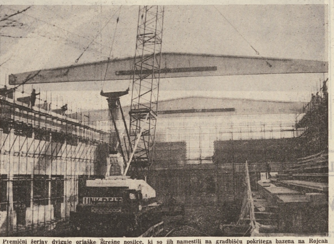
Prémicni žerjav dviguje orjaške štršne nosilce, ki so jih namestili na gradbišču pokritega bazena na Rojcah
