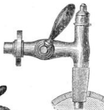
Podoba 72. Kolenasta cevna pipa (pasja glava) za sesalke s signalom (kadar je sod poln, pipa zažvižga).
