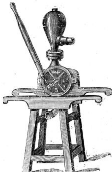
Podoba 66. Krilna sesalka za vino.
