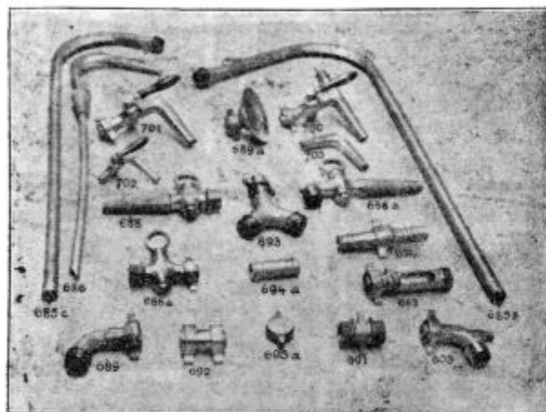
Podoba 68. Pritikline k vinskim sesalkam. Štev. 685b = polnatega; 585c = sesalna cev; 686 = nadanja natega; 688 = pipa za sod; 688a = ista vpognjena; 689 = kolenast holandec; 689 = vinski škropilnik; 591-693a = holandci; 700 = cevna pipa (pasja glava); 701 = ista z avtomatom; 702 = cevna pipa za gumijeve drobnejše cevi; 703 = cevno koleno; 683 = steklen holandec.
