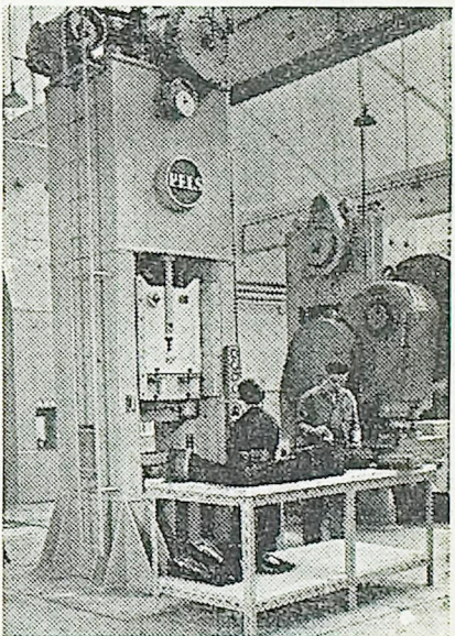
Stiskalnice z velikanskim pritiskom oblikujejo dele ogrodja in blatnike ter pločevinaste dele motornih koles, da ni potrebno nobeno obdelovanje več
