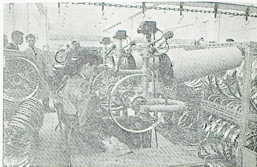
Kolo mora biti kar se da precizno centrirano. To opravljajo na posebnih strojih dekleta in žene — nekvalificirana delovna sila, kot večina zaposlenih v tovarni. Seveda je to mogoče le tam, kjer je uvedena proizvodnja po tekočem traku
