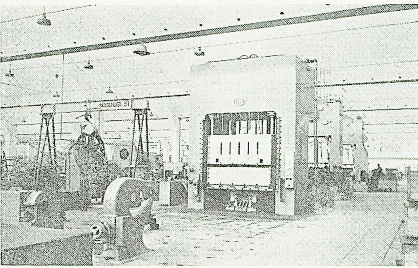
Mogočne stiskalnice do 600 ton pritiska oblikujejo okvire in gruge dele za motorna kolesa
