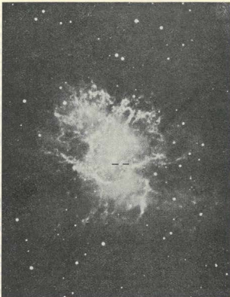
Rakova meglica. Črtici označujeta pulsar, ostanek osrednjega dela zvezde, ki je eksplodirala okrog leta 5550 pred Kr. Zaradi oddaljenosti pa je bila supernova vidna šele leta 1054 po Kr.
