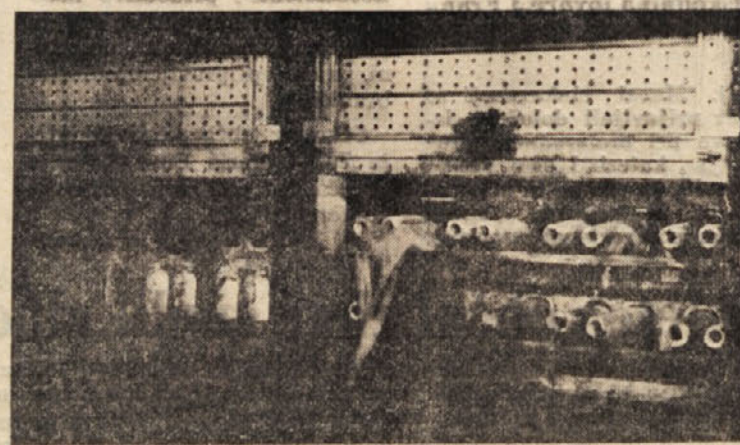
Nastavljanje predležev na retorte destilacijskih peči
