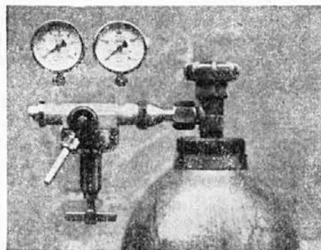
REDUCNI VENTIL »AGA-RUŠE« Z NAVZDOL OBRNENIM REGULIRNIM VIJAKOM.
