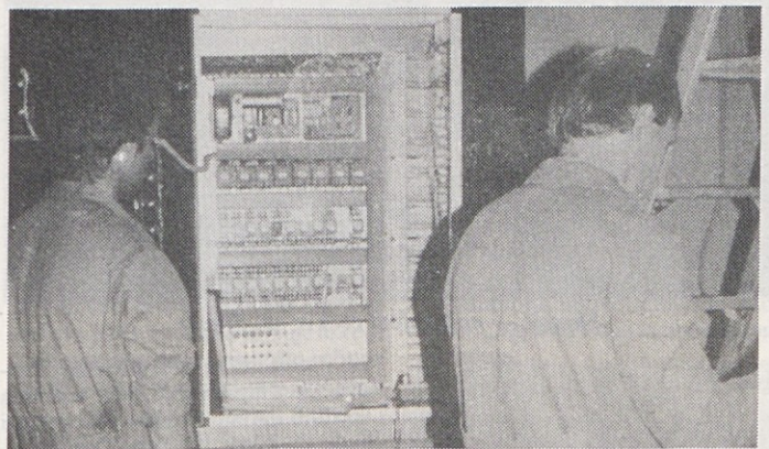
Za požarno varnost v čistilnici in mikalnici je velika pridobitev drugi del naprave za odkrivanje in javljanje požarov v transpornih cevovodih. Na fotografiji sta monterja Zarje iz Kamnika, ki opravljata zaključna dela.
