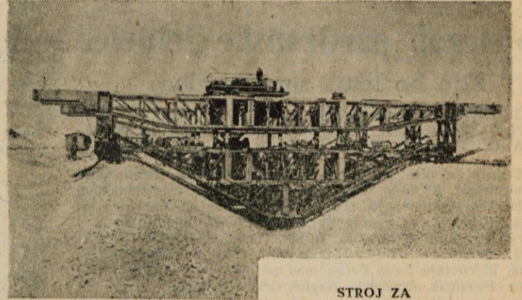
STROJ ZA BETONIRANJE JARKOV,
