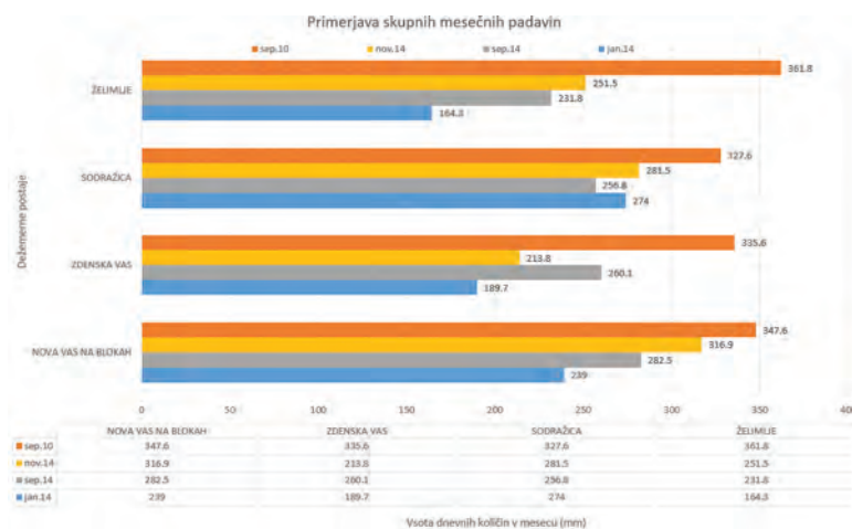
Graf 1: Skupne mesečne padavine
