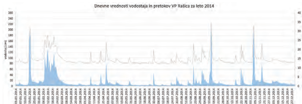
Graf 7: Dnevne vrednosti vodostajev in pretokov na VP Rašica za leto 2014
