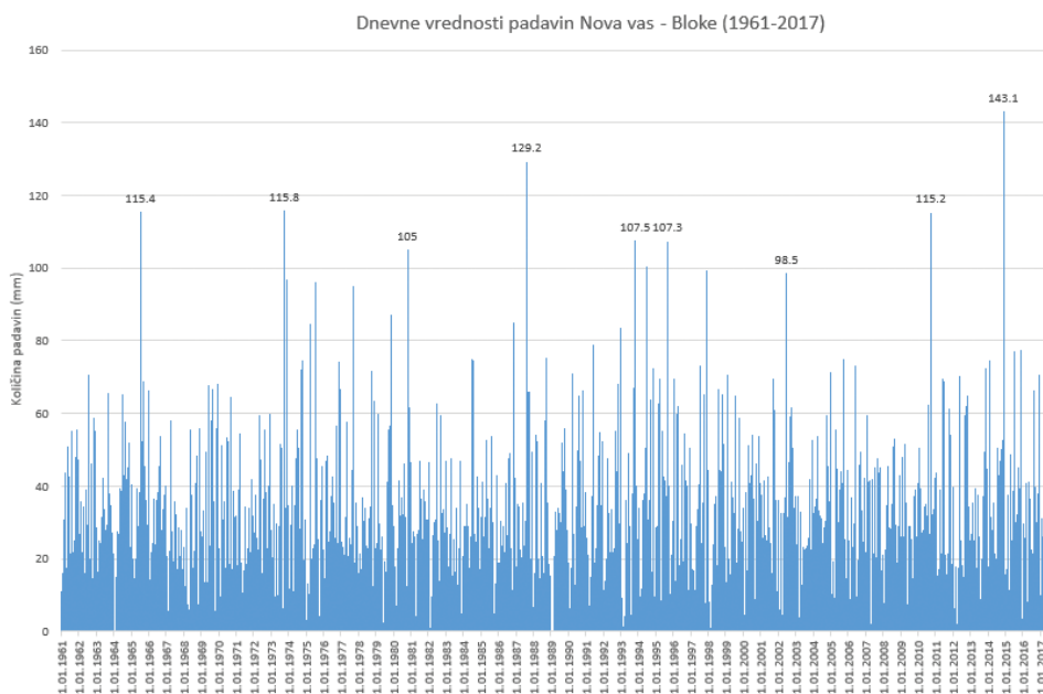
Graf 5: Dnevne vrednosti padavin za postajo Nova vas na Blokah
