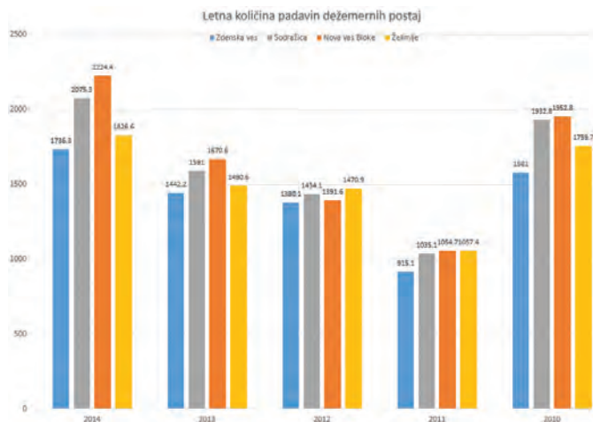
Graf 3: Letna količina padavin
