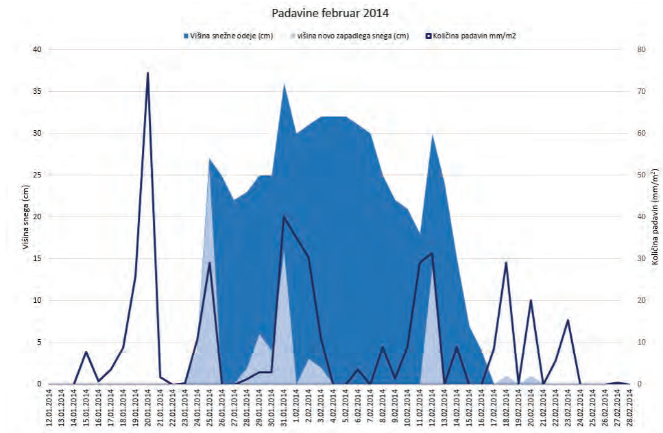
Graf 9: Padavine februar 2014
