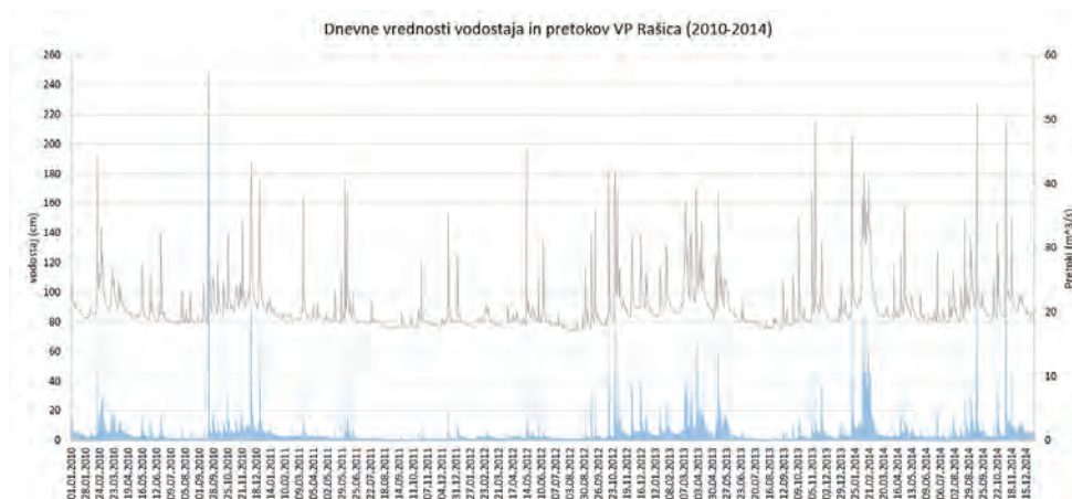
Graf 6: Dnevne vrednosti vodostaja in pretokov (2010-2014)
