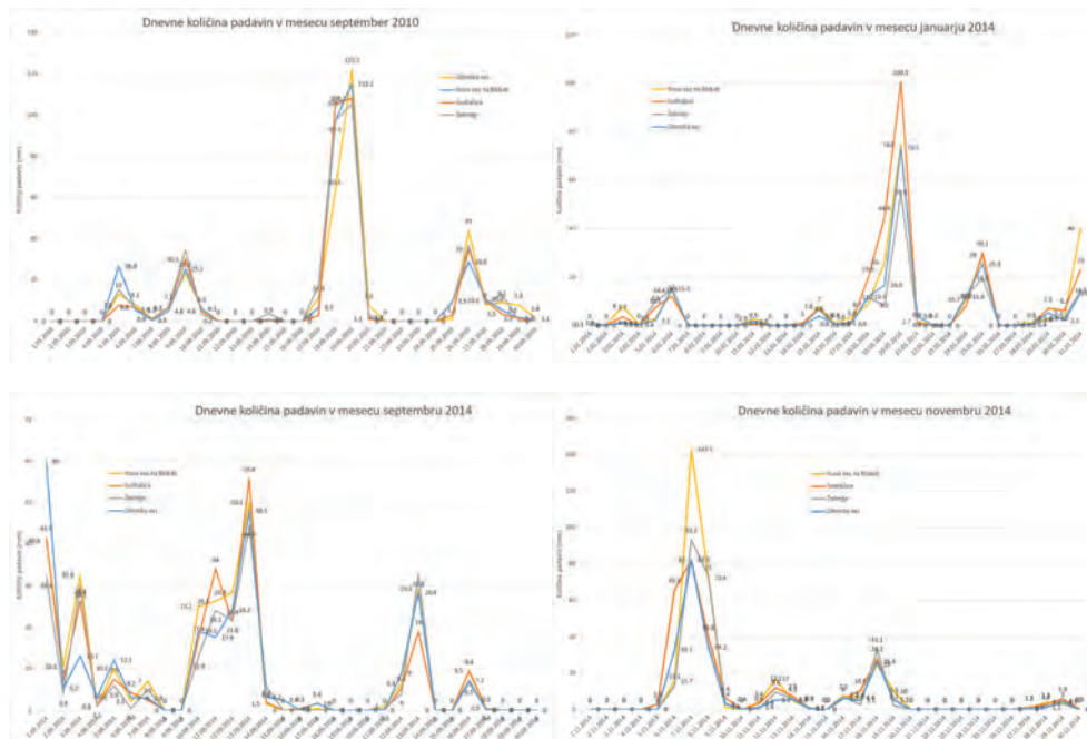
Graf 2: Dnevne količine padavin v času poplavnega dogodka
