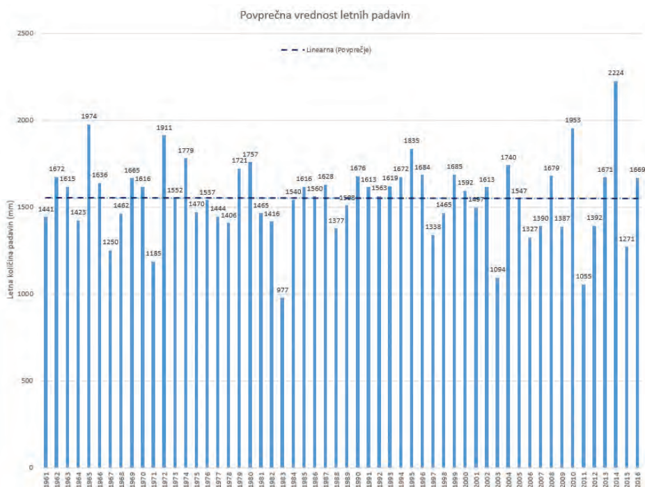
Graf 4: Letno povprečje padavin za postajo Nova vas na Blokah
