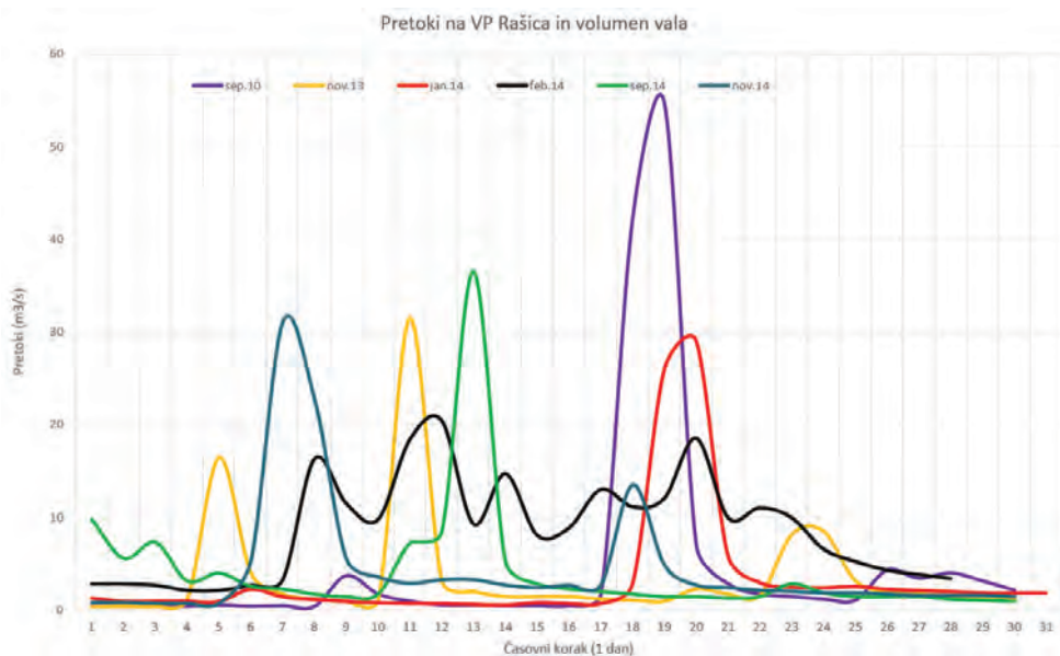
Graf 8: Graf pretokov za posamezne dogodke
