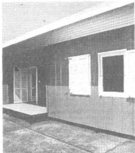
Prototip 90 kvadratnih metrov velike TRIMO-IKOR 83 stanovanjske hiše so si na obrtnem sejmu v Celju ogledali tudi Maks Klanšek, Aleš Ruch in Peter Vrhunc in se strinjali s predlogom, naj bi podoben prototip zgradbe postavili poskusno tudi na Barju.
