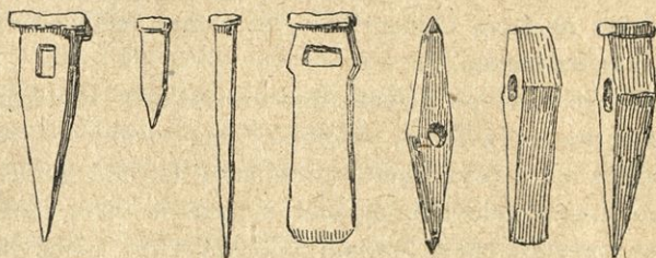
Obr. 40. Římské dolovací nářadí z Dacie (podle G. Téglláse).
