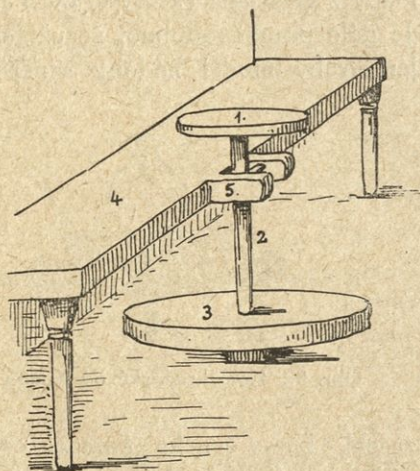
Obr. 94. Hrnčírský kruh huculský (Šuchevyč).
