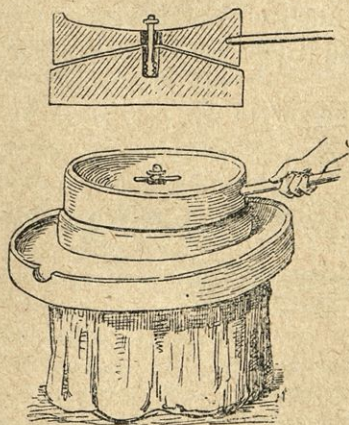
Obr. 25. Římský mlýnec ze Saalburgu. (podle L. Jacobiho.)
