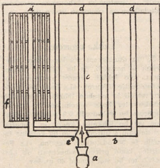
Prezračevališče na 3 kamrice: a) puhalnik, b) glavni sapnik, c) stranski sapnik, d) kamrice, e) zaporna vrata, f) mreža iz letev
