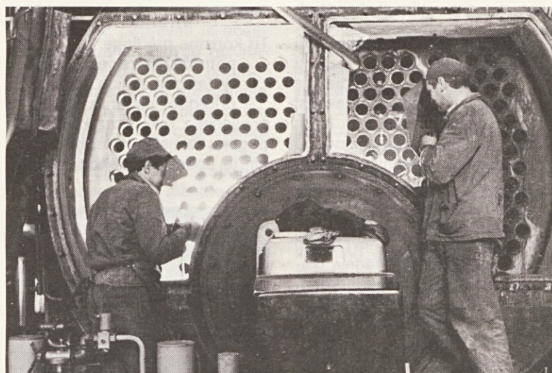
Obnovitev plamenišča na večjem kotlu
