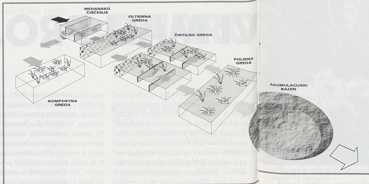
Schema rastlinske čistilne naprave z zbiranjem očiščene vode v kalu
