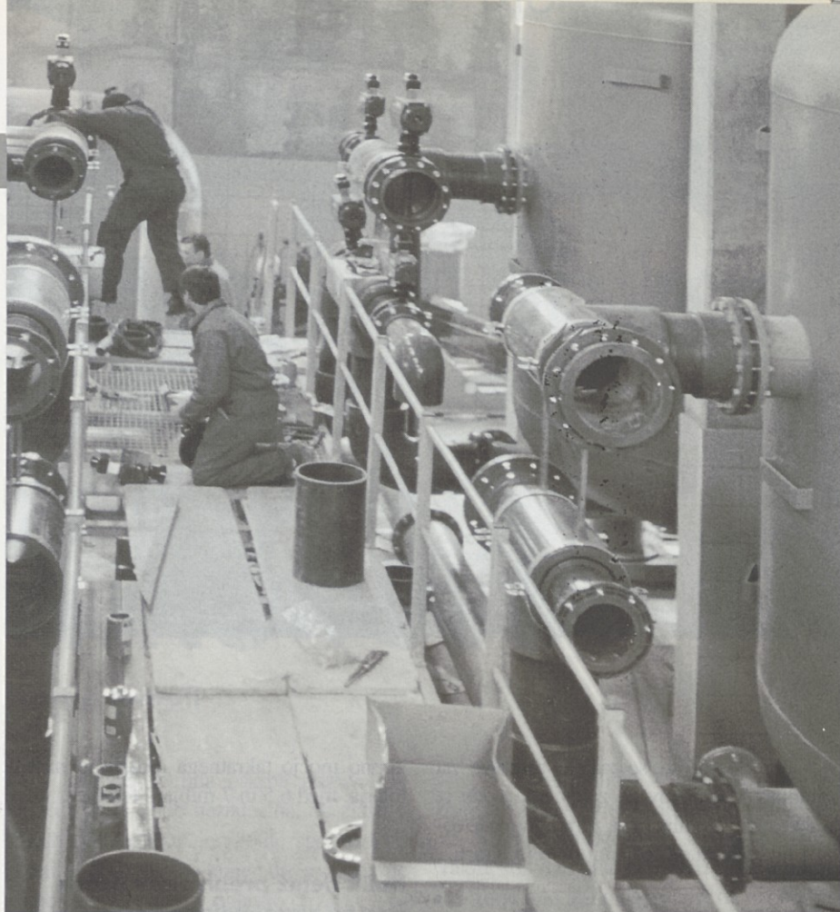
Montaža tehnologije za obdelavo surove vode.
